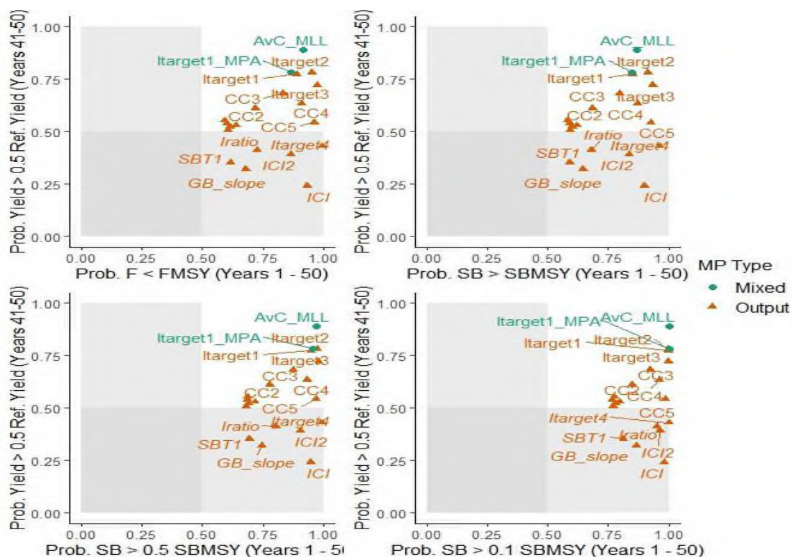
Рисунок 14 – Оценка эффективности стратегий управления при определении величины ОДУ стерляди в водных объектах Томской области с использованием программы DLMtool
