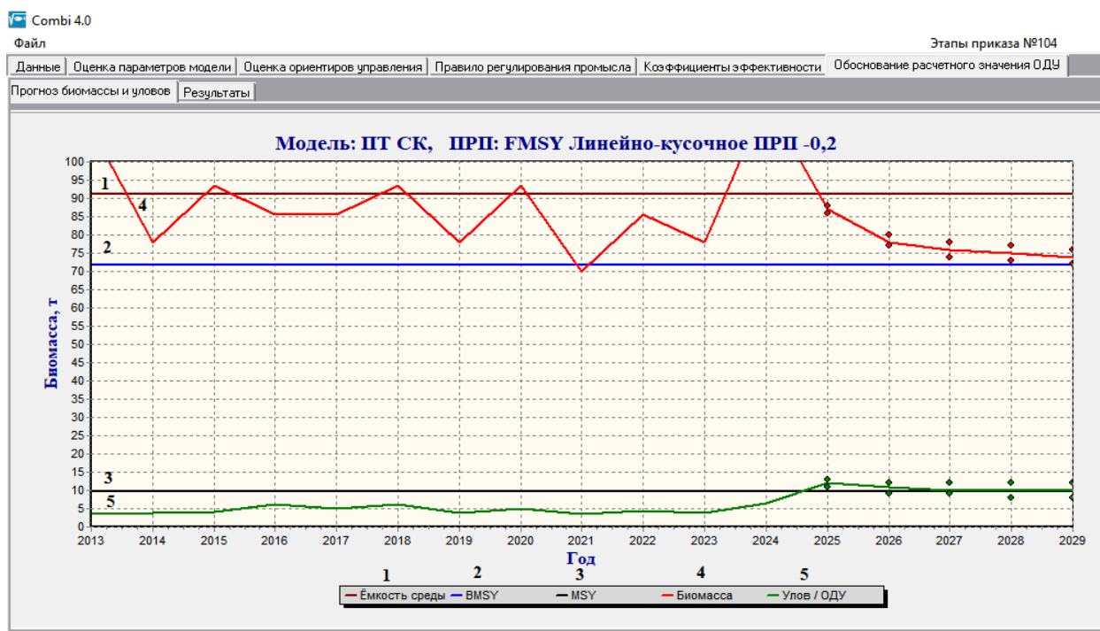
Рисунок 11 – Прогноз состояния биомассы и ОДУ стерляди в водных объектах Томской области на 2026–2029 гг. с использованием программы COMBI 4.0
