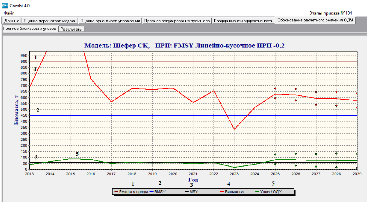
Рисунок 30 – Прогноз состояния биомассы и ОДУ пеляди на 2026–2029 гг. с использованием программы COMBI 4.0
