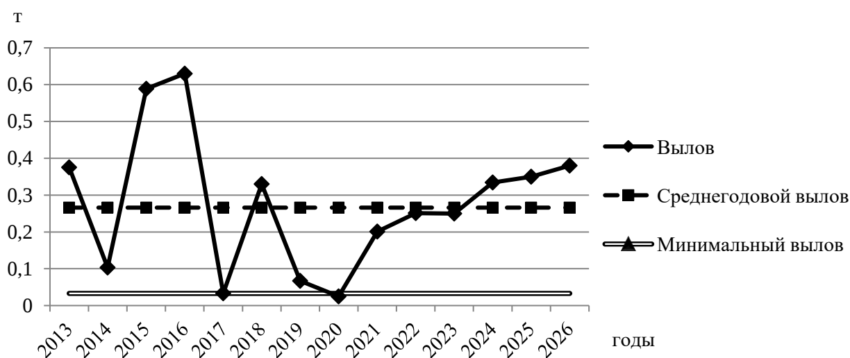
Рисунок 22 – Динамика вылова стада нельмы в р. Обь Томской области с 2013 г. по 2026 г. (данные за 2025–2026 гг. – прогнозируемые)
