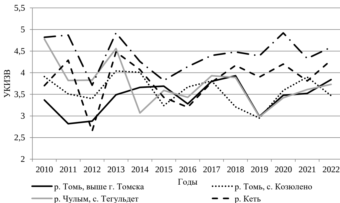
Рисунок 3 – Динамика УКИЗВ в притоках р. Обь в пределах Томской области (по данным Томского Центра по гидрометеорологии и мониторингу окружающей среды)
