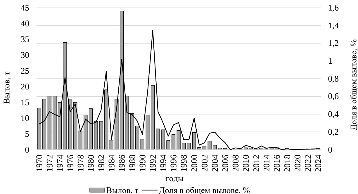
Рисунок 21 – Динамика уловов нельмы в Томской области (по официальным данным)
