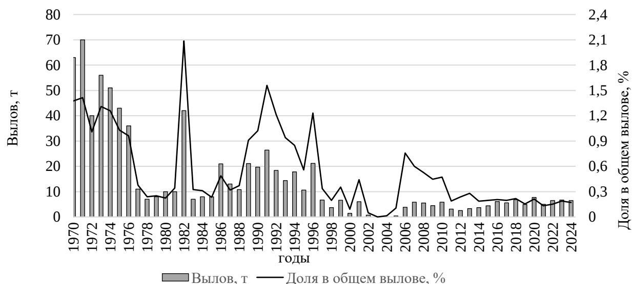
Рисунок 6 – Динамика уловов стерляди в Томской области (по официальным данным)
