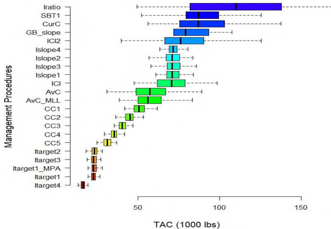
Рисунок 32 – Диапазон оценок ОДУ применяемых процедур управления к запасам пеляди в водных объектах Томской области с использованием программы DLMtool
