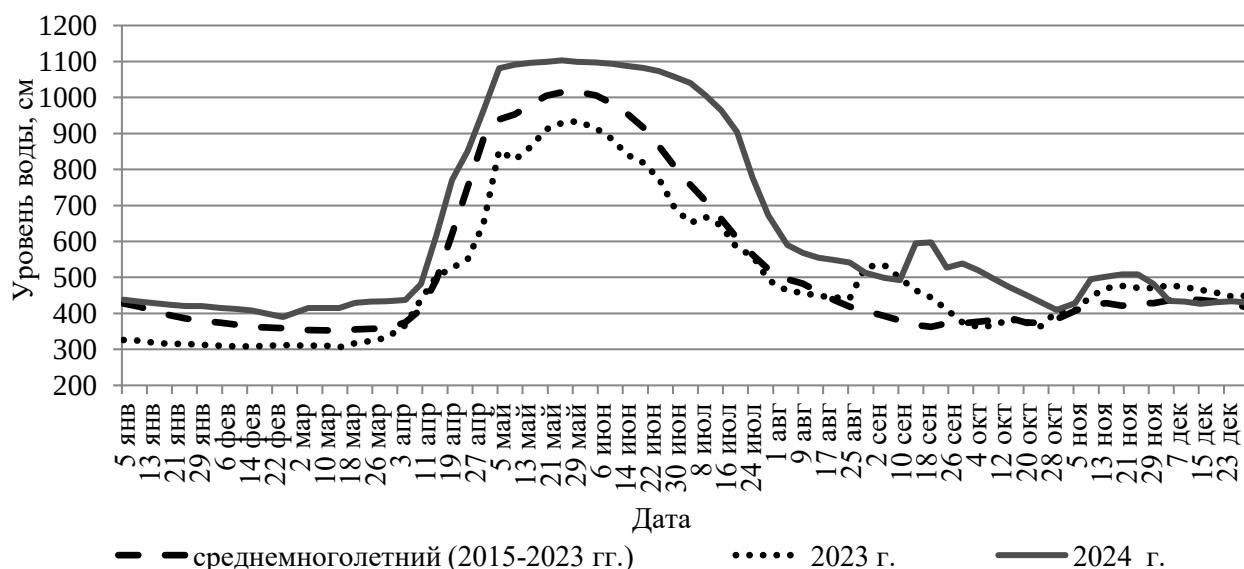
Рисунок 1 – Динамика уровня воды, Средняя Обь, 2015–2024 гг. (гидропост в пгт. Каргасок)
