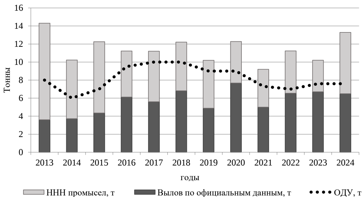
Рисунок 7 – Вылов и ОДУ стерляди в Томской области за период 2013-2024 гг., т
