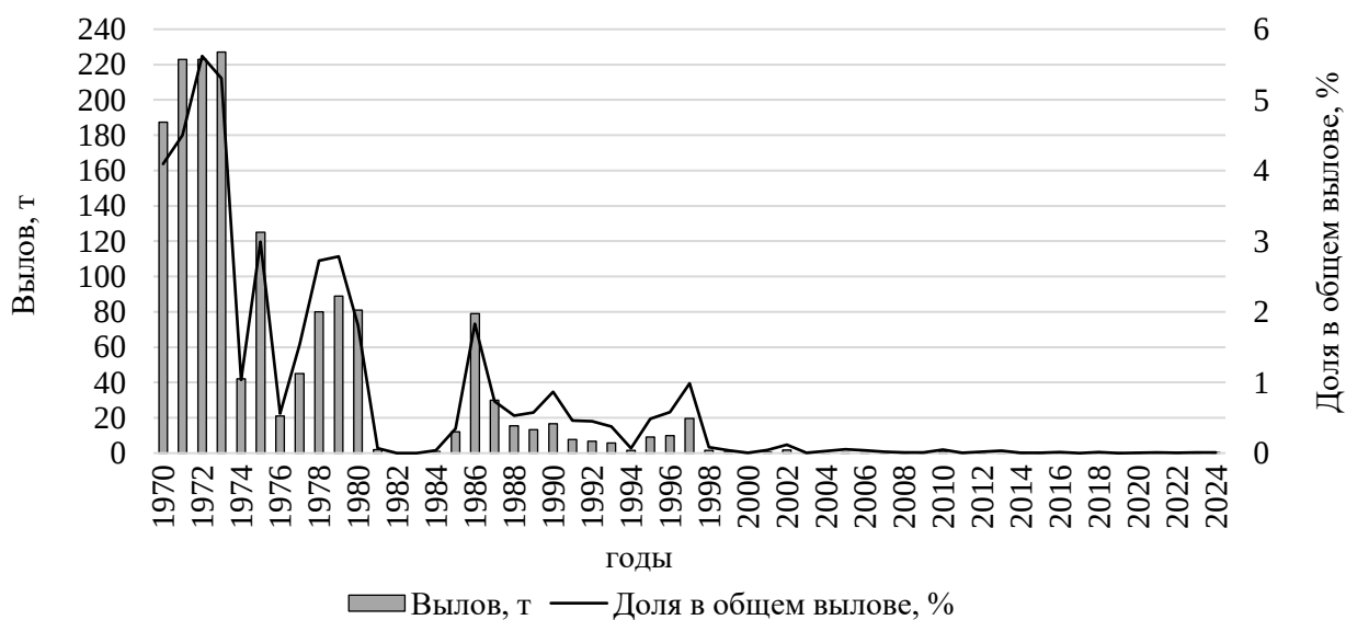
Рисунок 16 – Динамика уловов муксуна в Томской области (по официальным данным)
