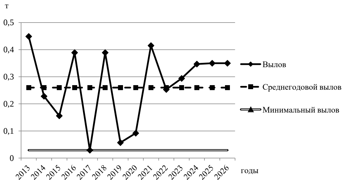
Рисунок 17 – Динамика вылова муксуна в р. Обь Томской области с 2013 г. по 2026 г. (данные за 2025–2026 гг. – прогнозируемые)
