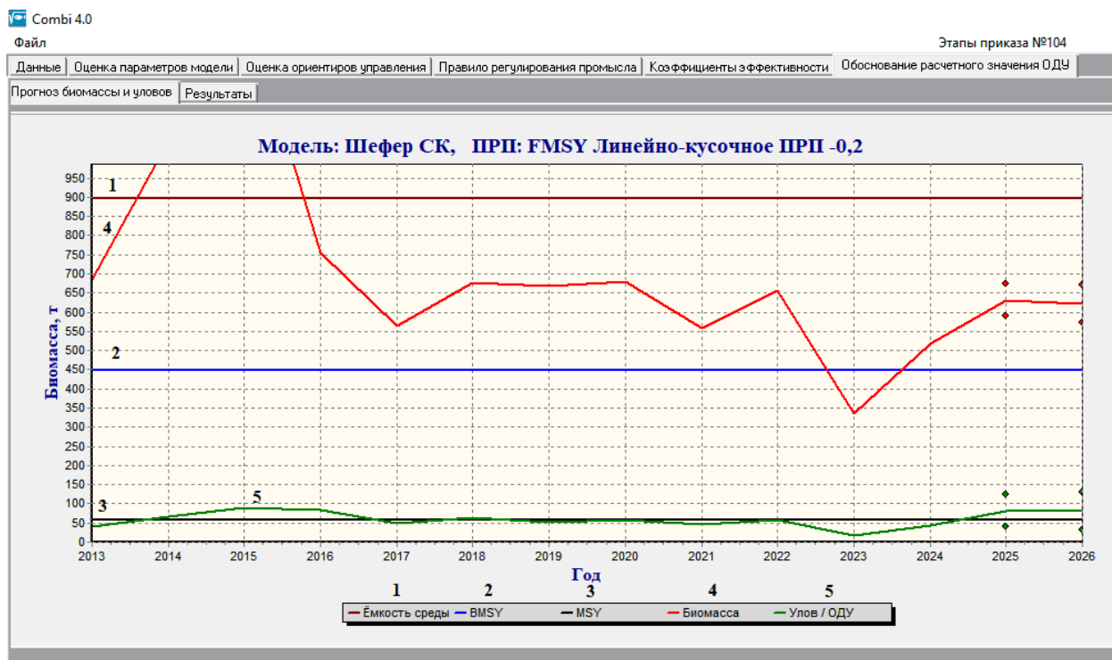
Рисунок 28 – Прогноз биомассы и ОДУ пеляди в водных объектах Томской области на 2025–2026 гг. с использованием программы COMBI 4.0
